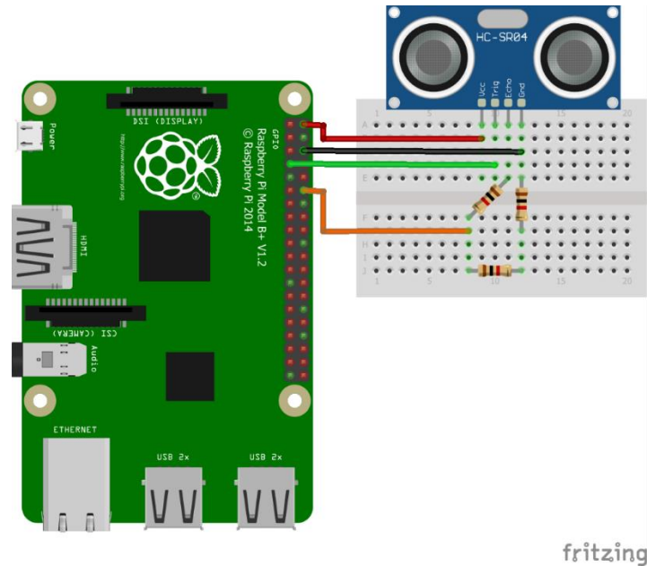
Figura 10 Diagrama esquemático do circuito com sensor de distância ligado aos pinos GPIO.
