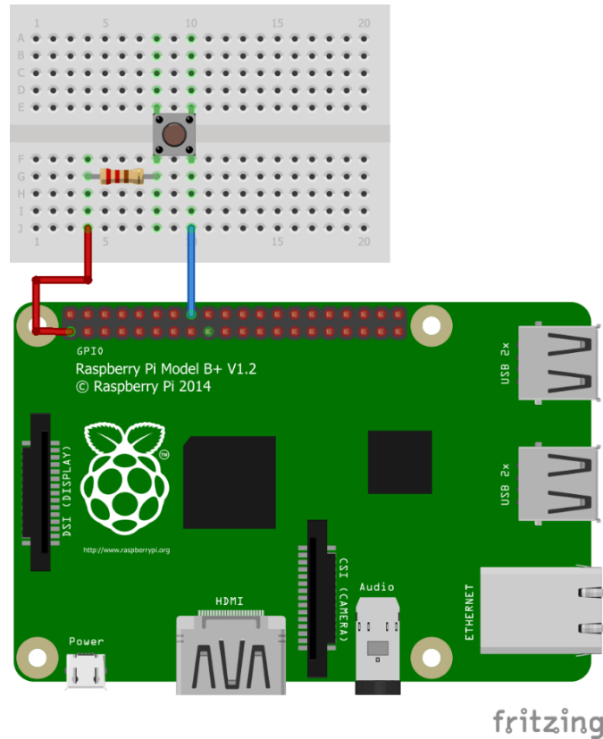
Figura 7 Ligação de um botão de pressão à GPIO utilizando uma placa de ensaio e dois cabos de ligação.
