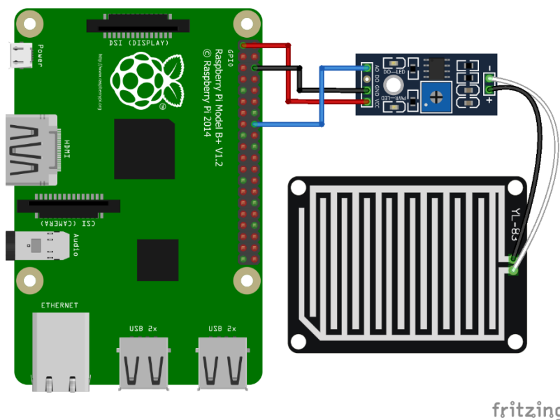
Figura 13 Esquema do sensor detetor de chuva ligado aos pinos GPIO da Raspberry Pi.
