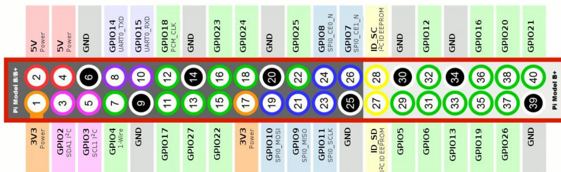
Figura 5 Pinos da GPIO Raspberry Pi
