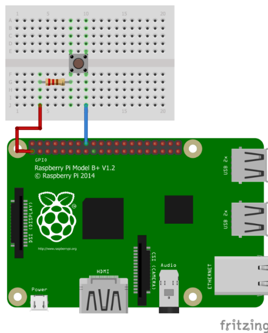
Figura 4 Ligação de um botão de pressão à GPIO utilizando uma placa de ensaio e dois cabos de ligação.
